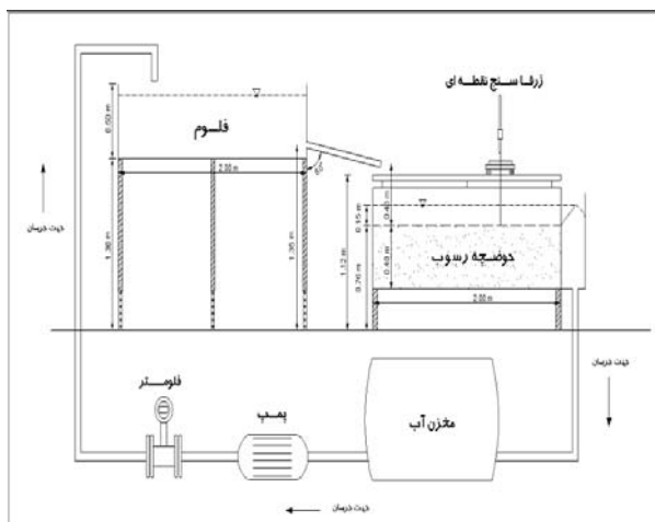
شکل ۳: شکل شماتیک از تجهیزات آزمایشگاه (جت ریزشی)
