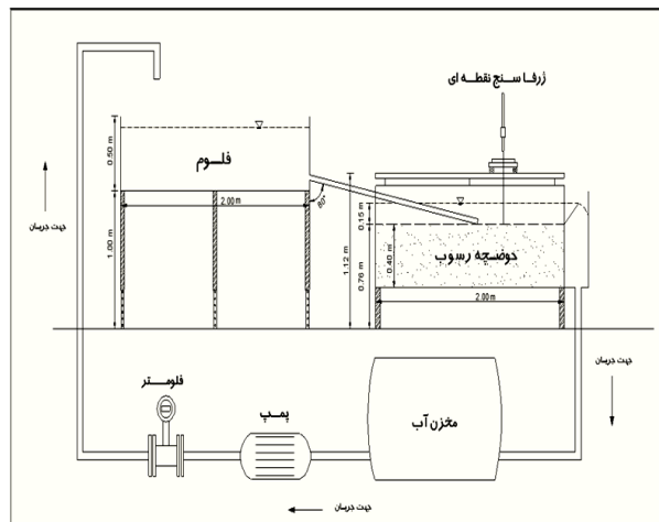
شکل ۲: شکل شماتیک از تجهیزات آزمایشگاه (جت مستغرق)
