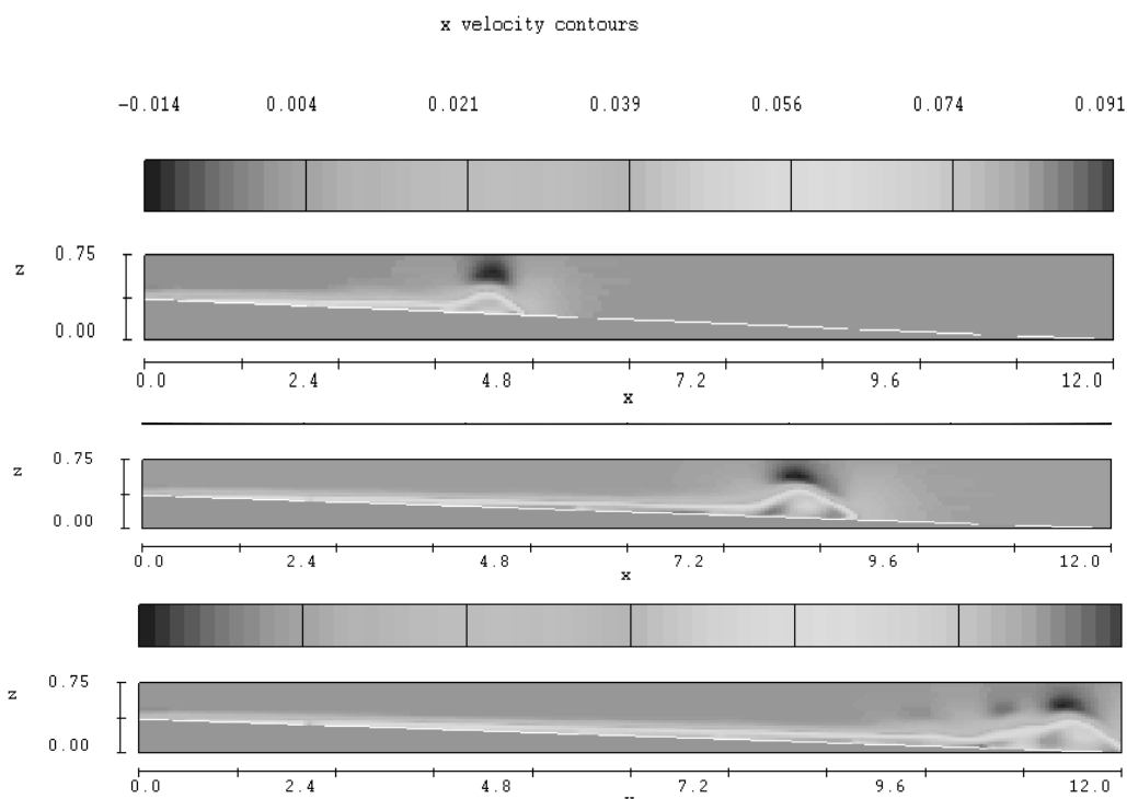
شکل ۴- الگوی جریان چگال شبیه سازی شده در زمانهای مختلف، شیب کانال ۳ درصد، غلظت ۱ درصد و دبی ۳۰ لیتر بر دقیقه
