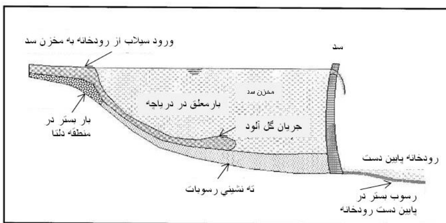
شکل ۱- یک جریان گل‌آلود پیوسته در مخزن سد [۳]
