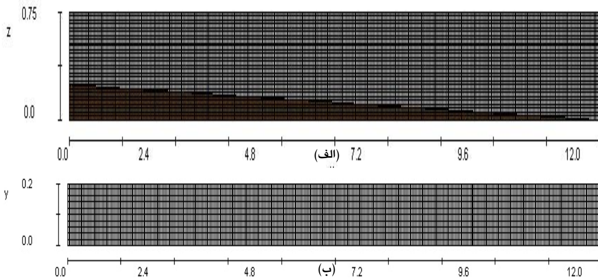
شکل ۳- ترسیم شبکه جریان (الف- جهت X-Z) (ب- جهت X-Y)
