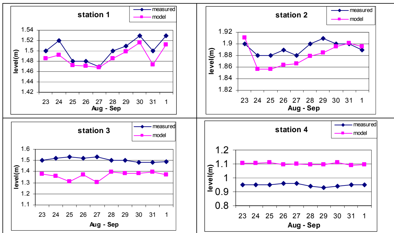
شکل ۲: نتایج کالیبراسیون مدل هیدرودینامیک در نواحی شرقی (ایستگاه ۱)، غربی (ایستگاه ۱۱) در لاگون انزلی و ایستگاه ۱۲ در ناحیه سیاه کشیم) و مرکزی (ایستگاه ۱۵) تالاب انزلی در ماه آگوست
